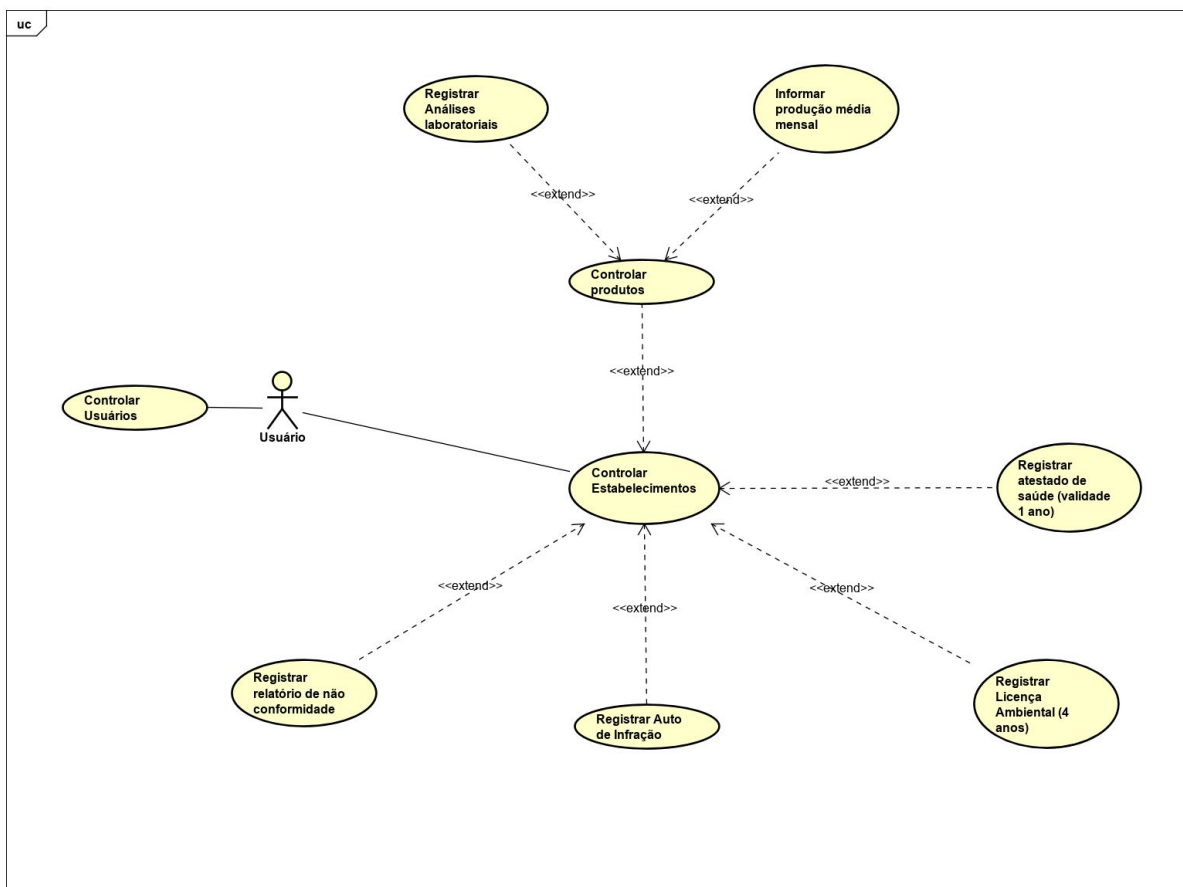
Figura 6: Diagrama de casos de uso SIMSIM. Elaborado pelo Autor
