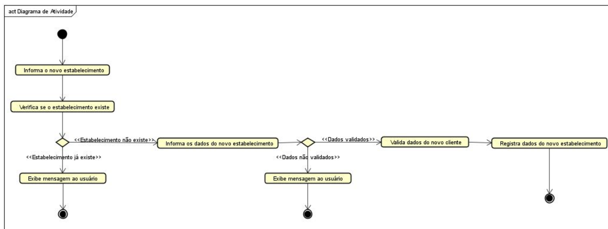
Figura 9: Diagrama de atividades SIMSIM. Elaborado pelo autor.
