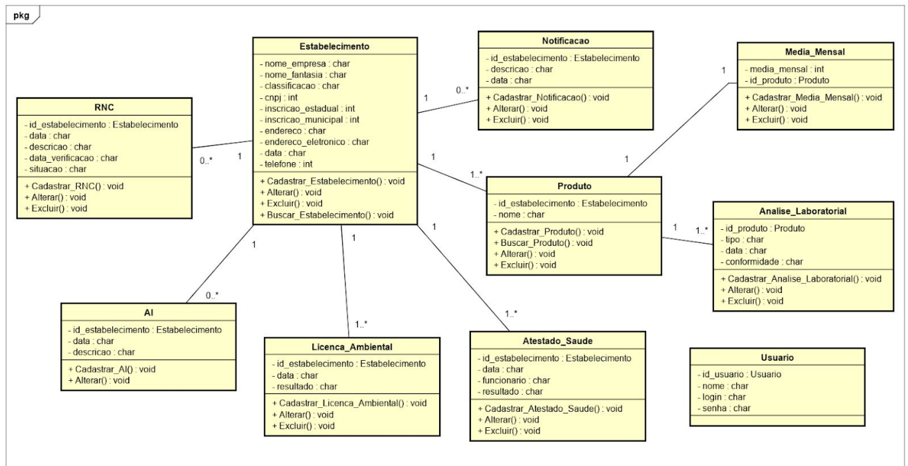
Figura 7: Diagrama de classes SIMSIM. Elaborado pelo Autor
