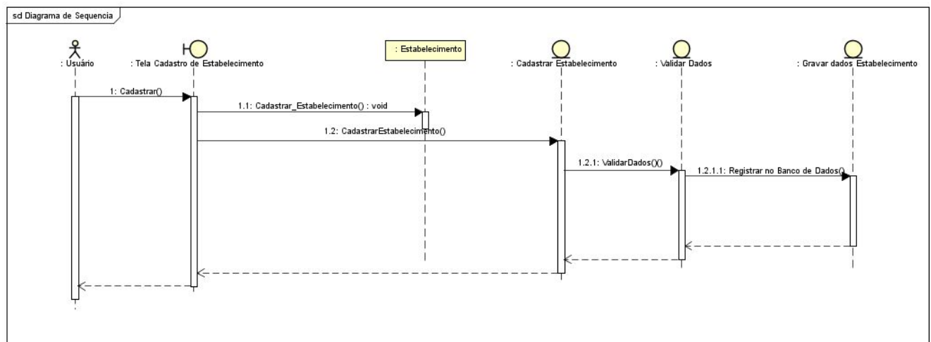
Figura 8: Diagrama de sequência SIMSIM. Elaborado pelo autor.
